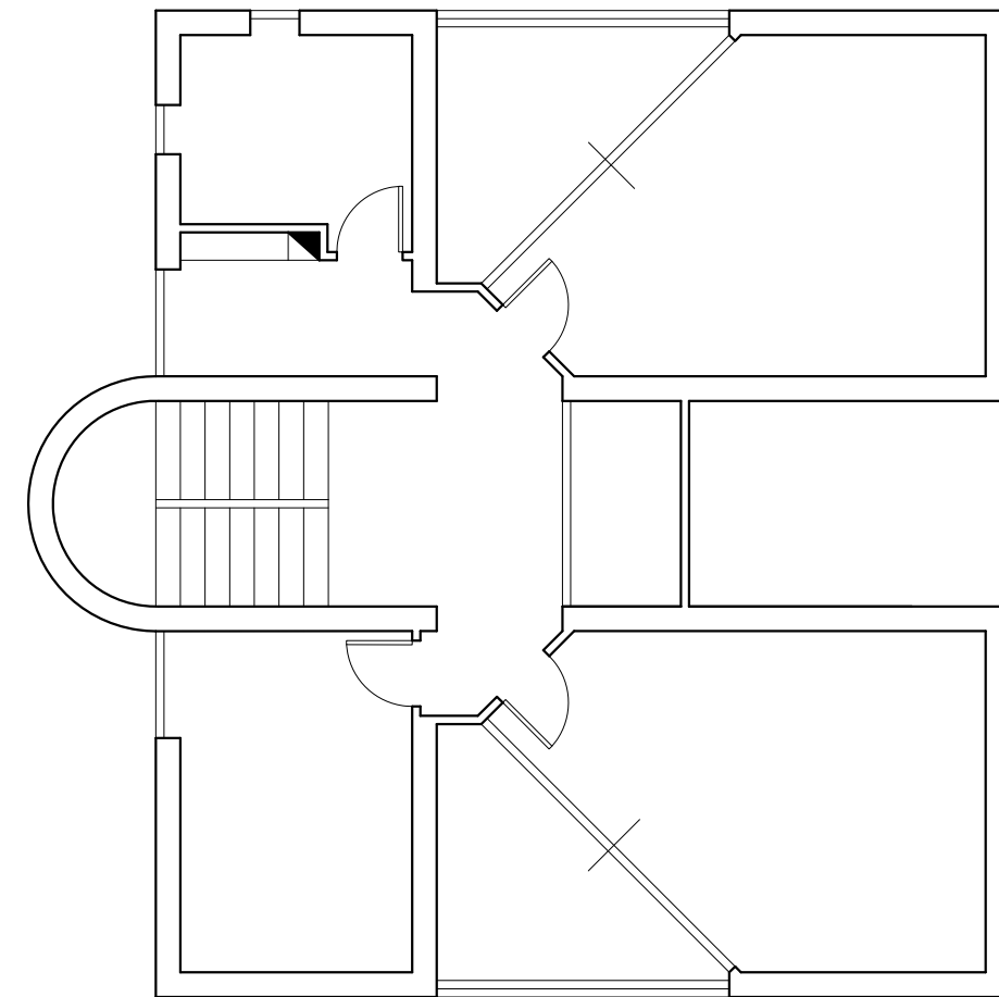
PIANO SECONDO
